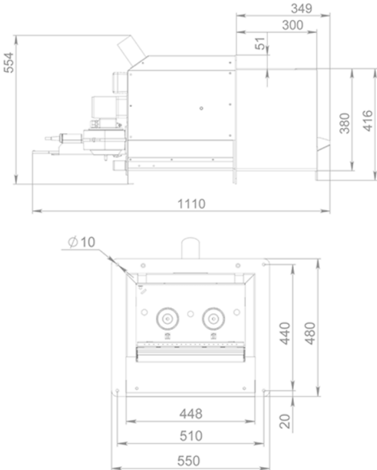
Рис. 1. Габаритные и присоединительные размеры горелки.
